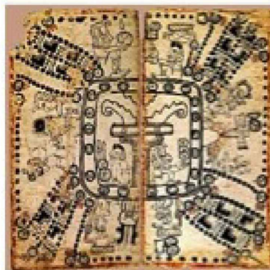
(c) Códice Madrid f. 75 y 76. Maya Clásico
